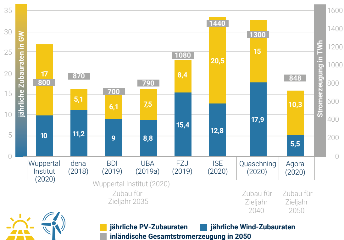
100 % EE – Überblick über Zubauraten und Gesamtstromerzeugung
